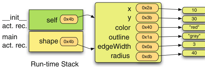
Fig. 7.3 A circle object
